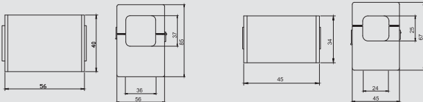
Teknik Resim Technical Drawing
