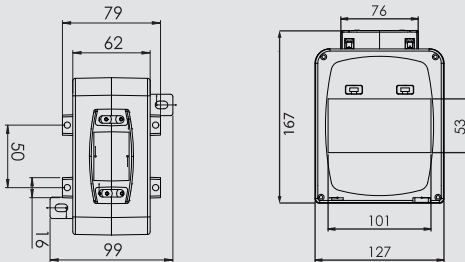
Teknik Resim Technical Drawing
