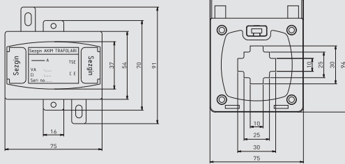
Teknik Resim Technical Drawing
