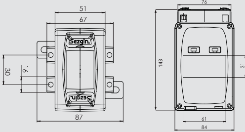
Teknik Resim Technical Drawing
