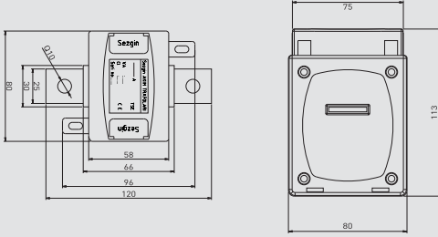
Teknik Resim Technical Drawing
